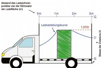
Lastenverteilungsplan für einen Kleintransporter mit einer zulässigen Gesamtmasse bis 3,5 t.
